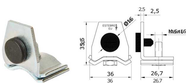
Door stop Code: 303-309
